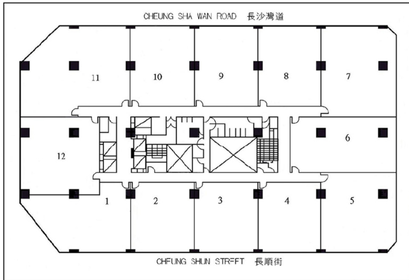
TYPICAL FLOOR PLAN OF TOWER 2, CHEUNG SHA WAN PLAZA 長沙灣廣場第二期標準平面圖
